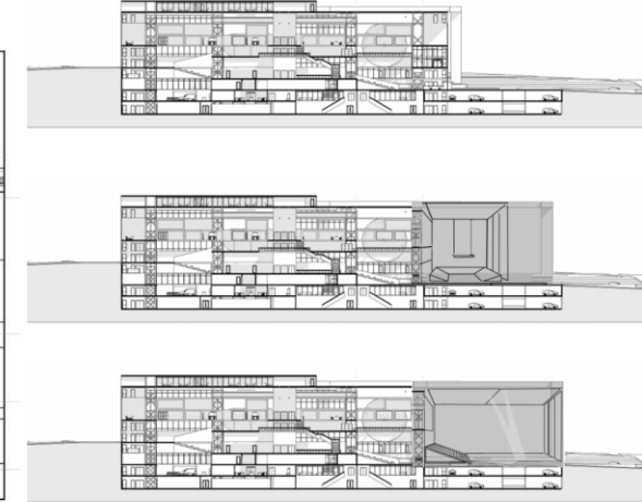
Kayar cephe kesitleri
